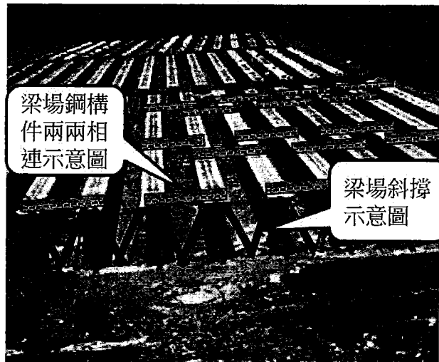
圖 6 梁場妥善固定預鑄預力 I 型梁
