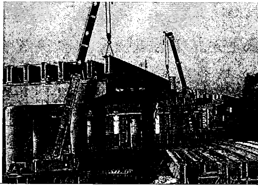
照片 9：預力梁之預鑄與吊放作業
