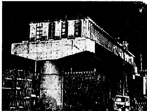
圖 8 端隔梁現場施工圖
